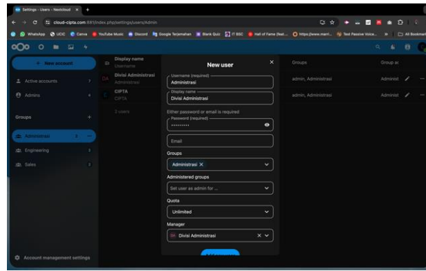
Gambar 11. Proses Penambahan Users
