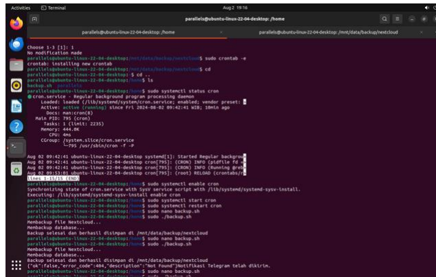
Gambar 14. Proses Konfigurasi Crontab
