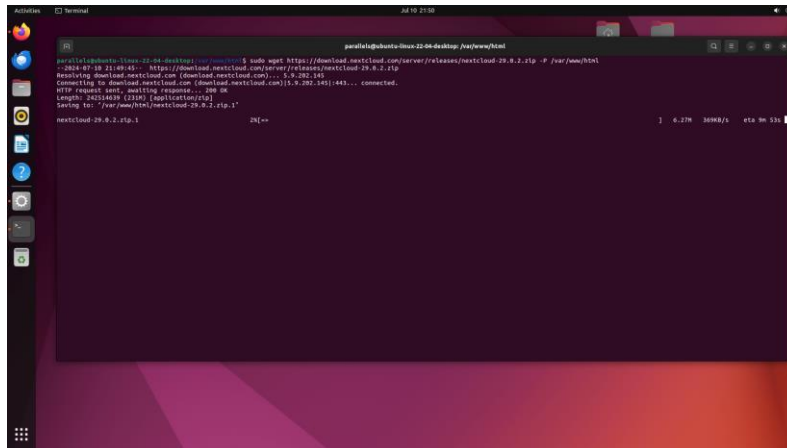
Gambar 2. Proses Installasi Ekstensi dan Nextcloud di Parallel Ubuntu
