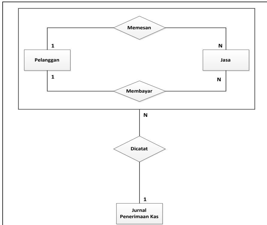
Gambar 3. ERD Sistem Akuntansi Penerimaan Kas
