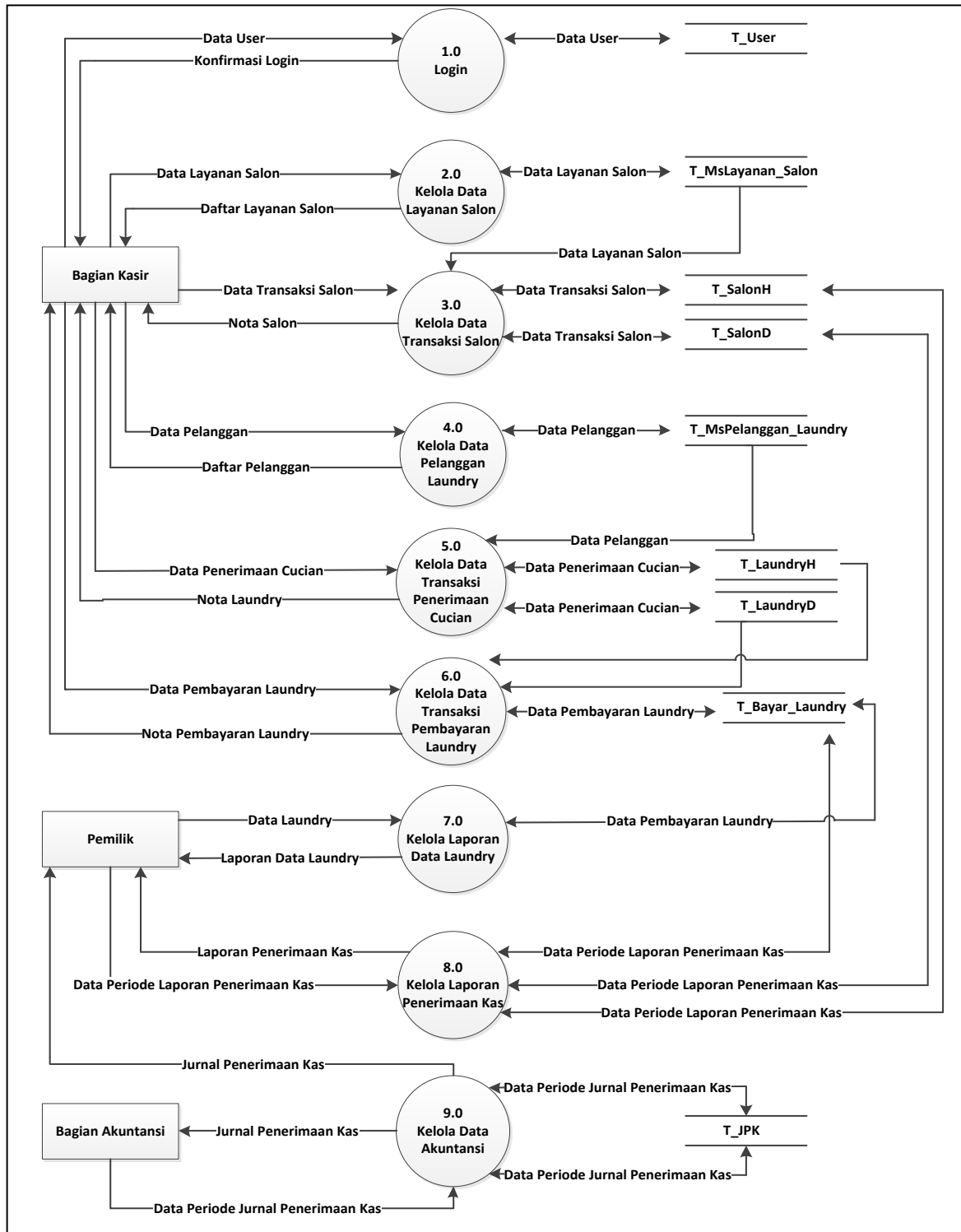
Gambar 2. DFD Level 0 Sistem Akuntansi Penerimaan Kas
