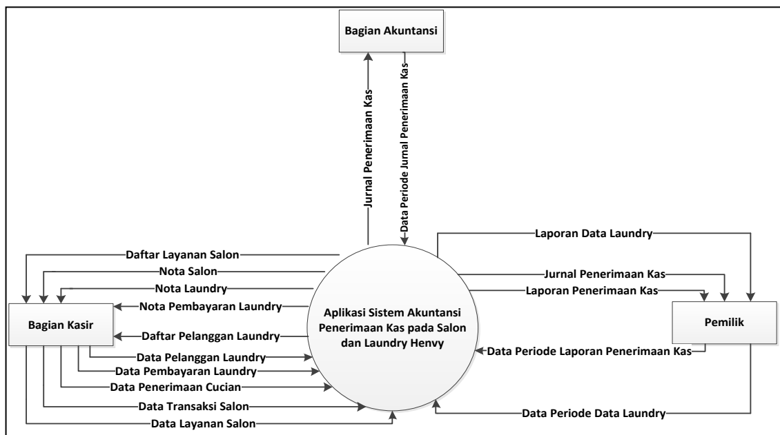
Gambar 1. Diagram Konteks
